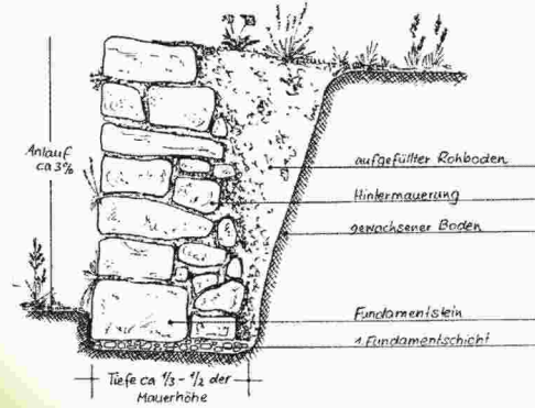
Schnitt durch eine Trockenmauer (Maueraufbau)
