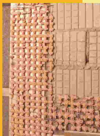
Überspannen von verschiedenen Materialien mit Ziegelgewebe zur Bewehrung des Lehmputzes
